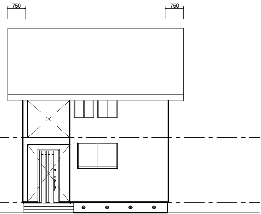
西立面図
