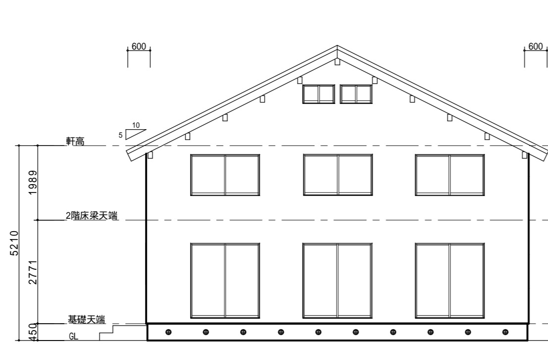
南立面図
