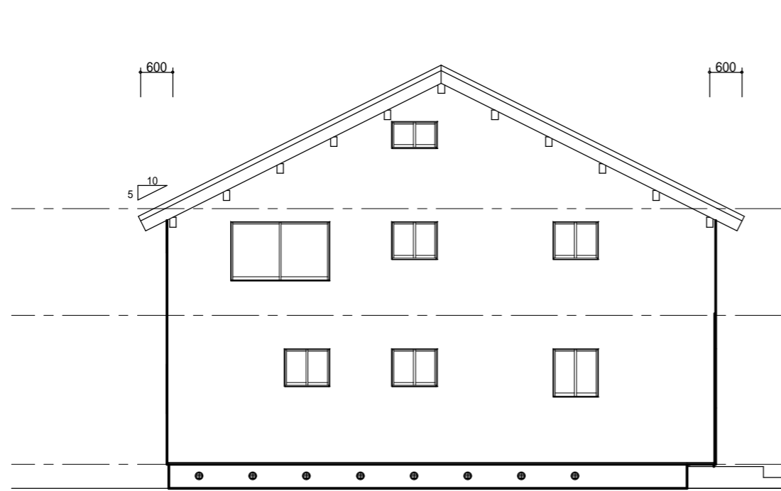
北立面図
